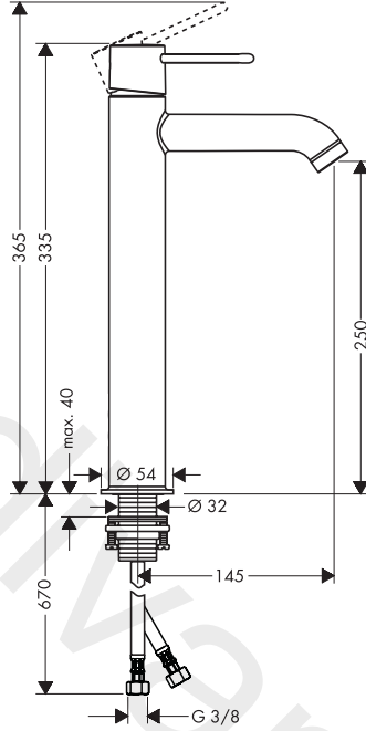
AXOR Uno 2 38027000
