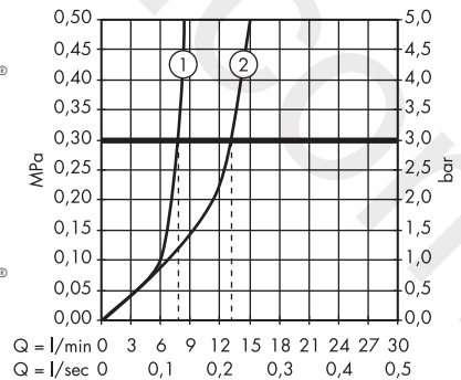
AXOR Uno 2 38210000
